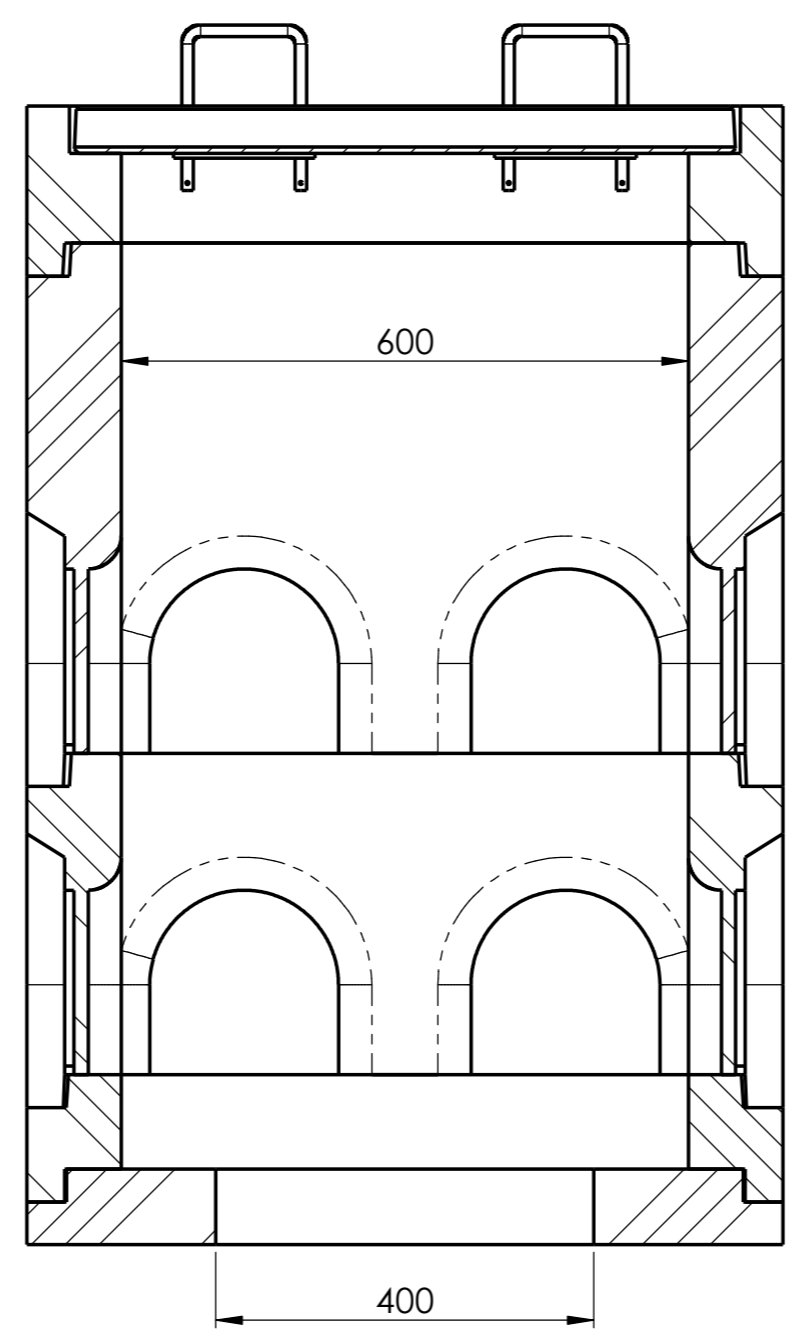
F-F (1 : 8)
