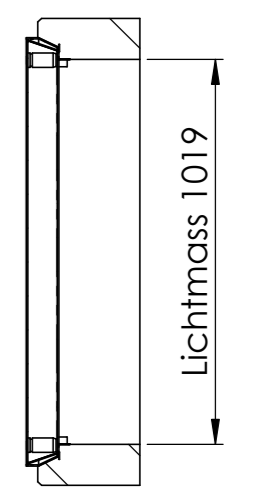
SCHNITT B-B MABSTAB 1 : 20
