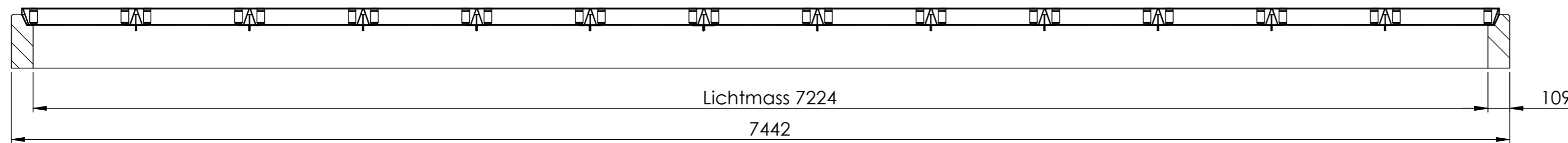
SCHNITT A-A MABSTAB 1 : 20
