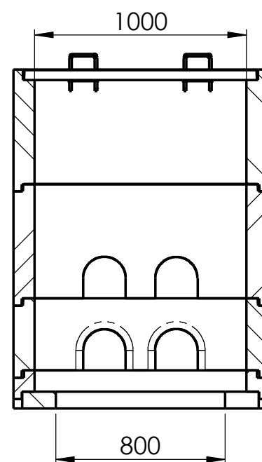
H-I (1 : 25)
