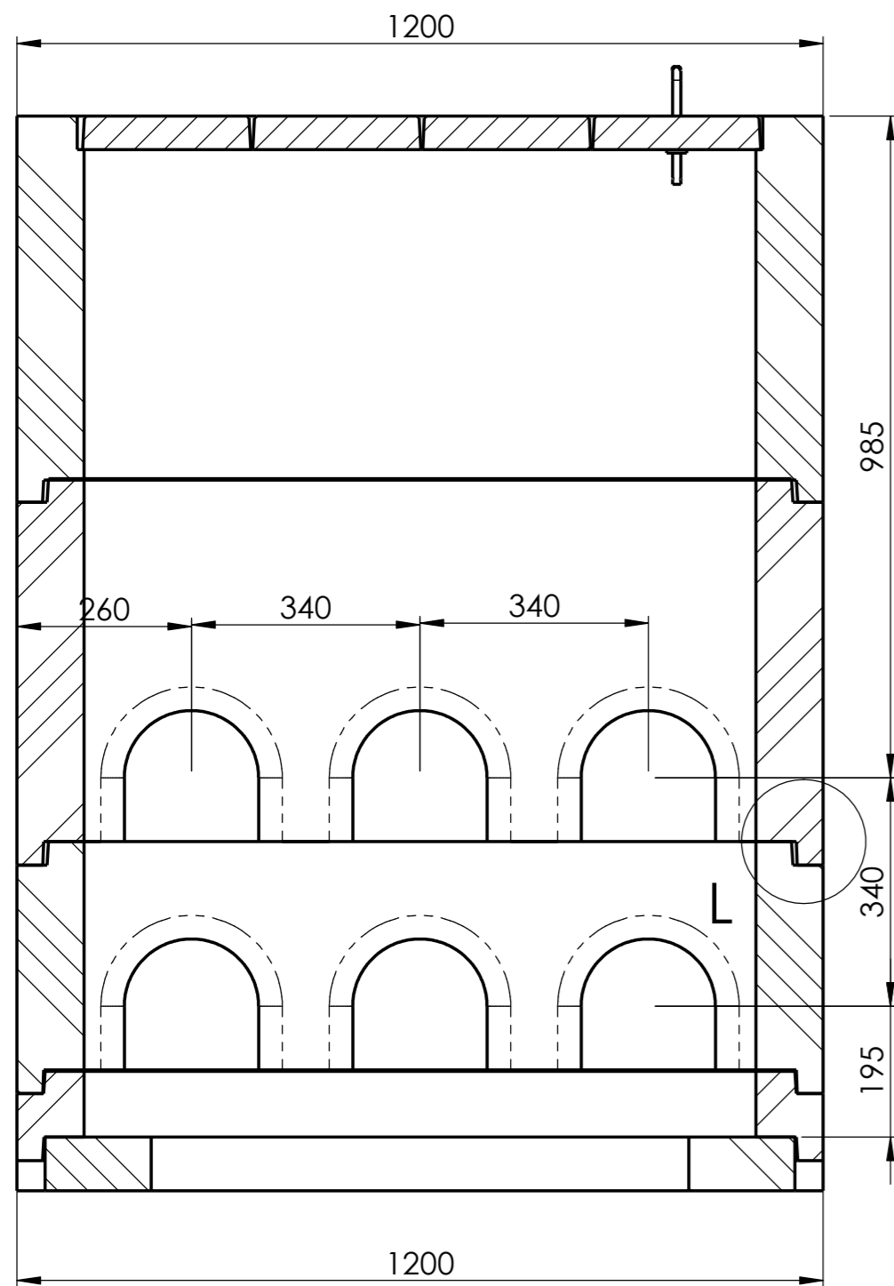
F-F (1 : 10)
