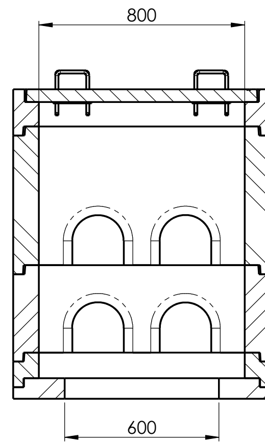
F-F (1 : 15)
