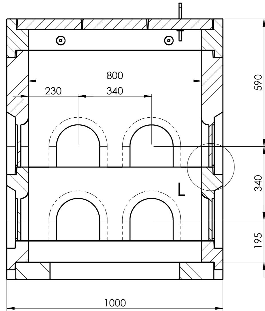
F-F (1 : 10)
