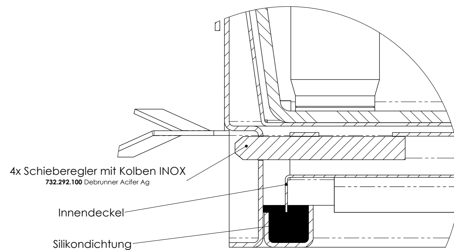
DETAIL c MAßSTAB 1 : 1
