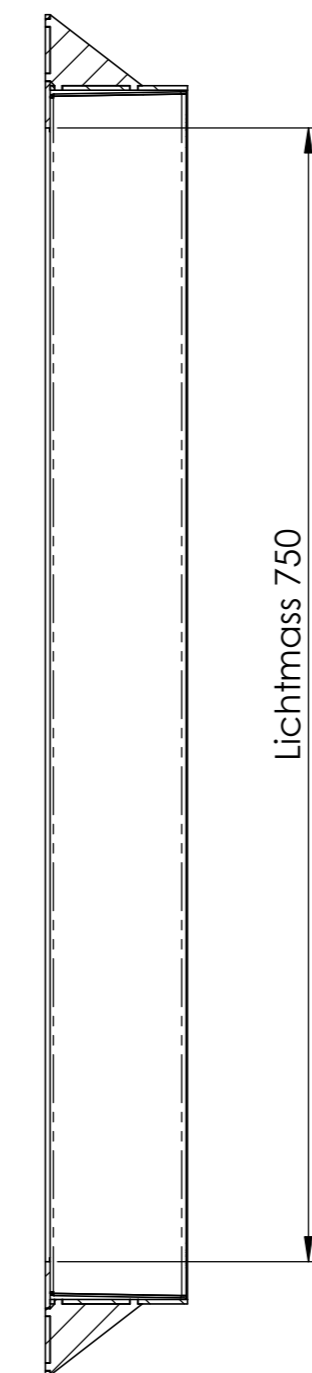
SCHNITT B-B MABSTAB 1 : 5
